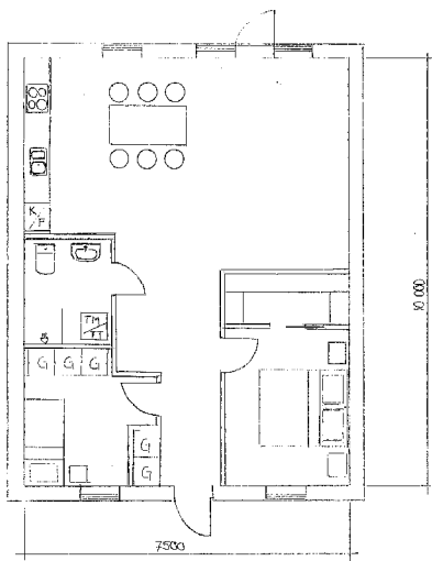
Ritning på en marklägenhet
